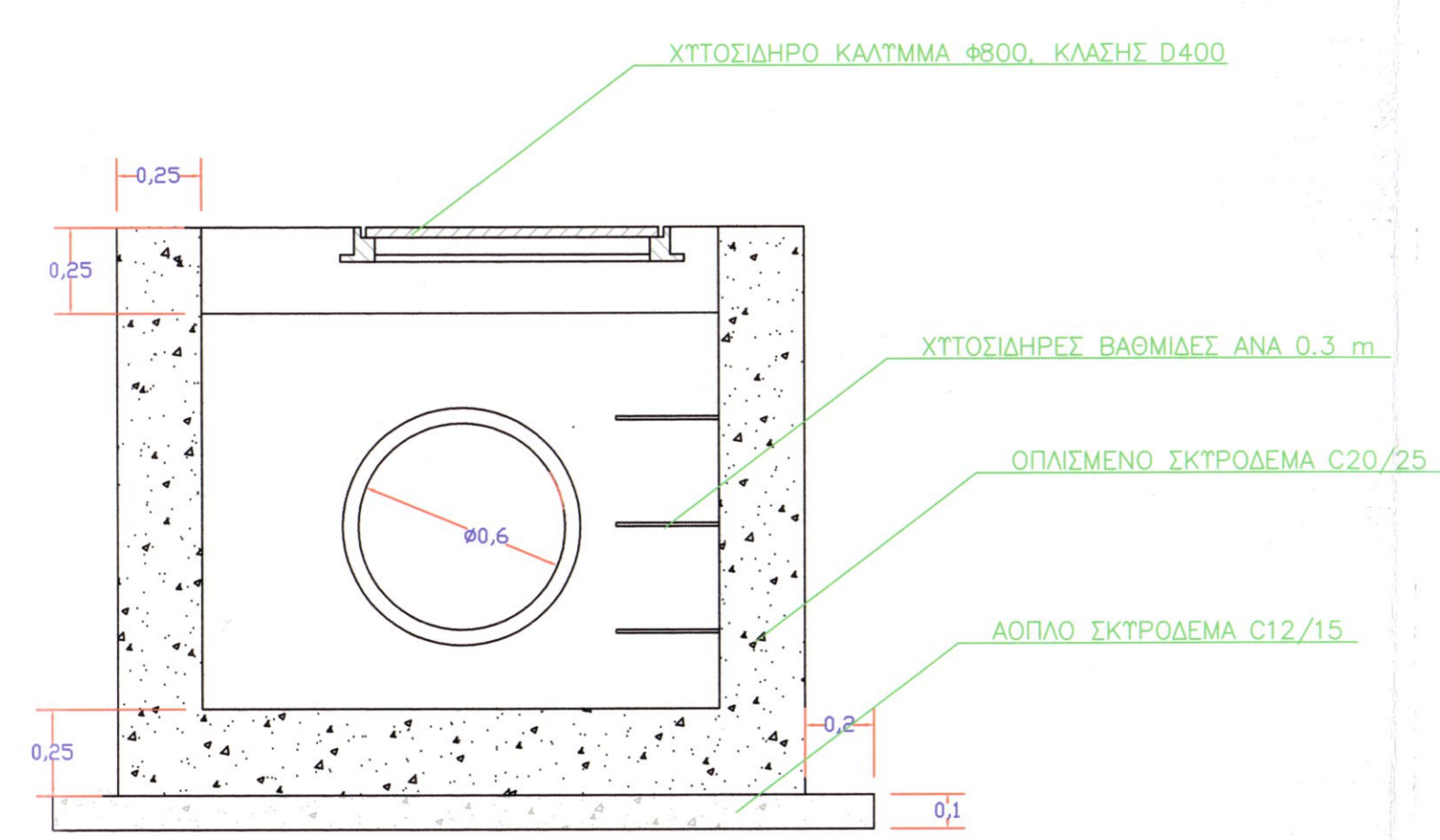
ΤΥΠΙΚΟ ΦΡΕΑΤΙΟ ΔΙΚΤΥΟΥ ΟΜΒΡΙΩΝ ΥΔΑΤΩΝ ΓΙΑ ΣΩΛΗΝΑ D600
