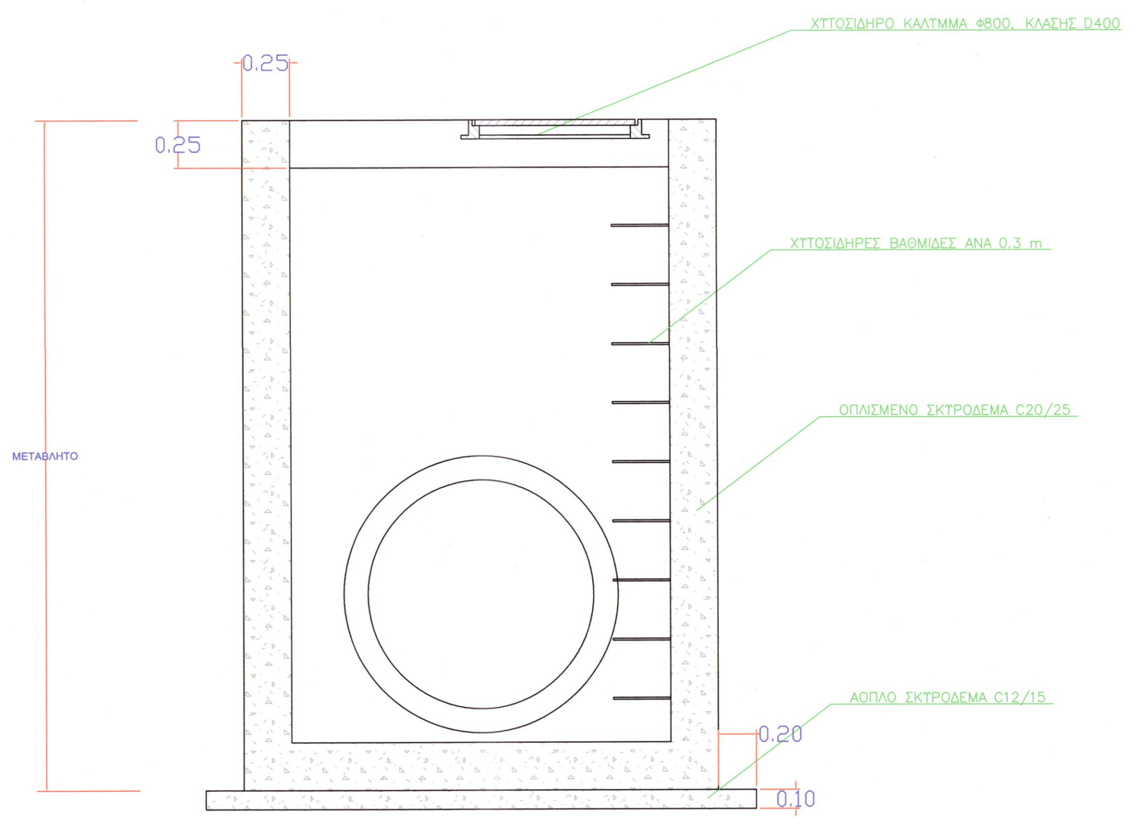
ΤΥΠΙΚΟ ΦΡΕΑΤΙΟ ΔΙΚΤΥΟΥ ΟΜΒΡΙΩΝ ΥΔΑΤΩΝ ΓΙΑ ΣΩΛΗΝΑ D1200
