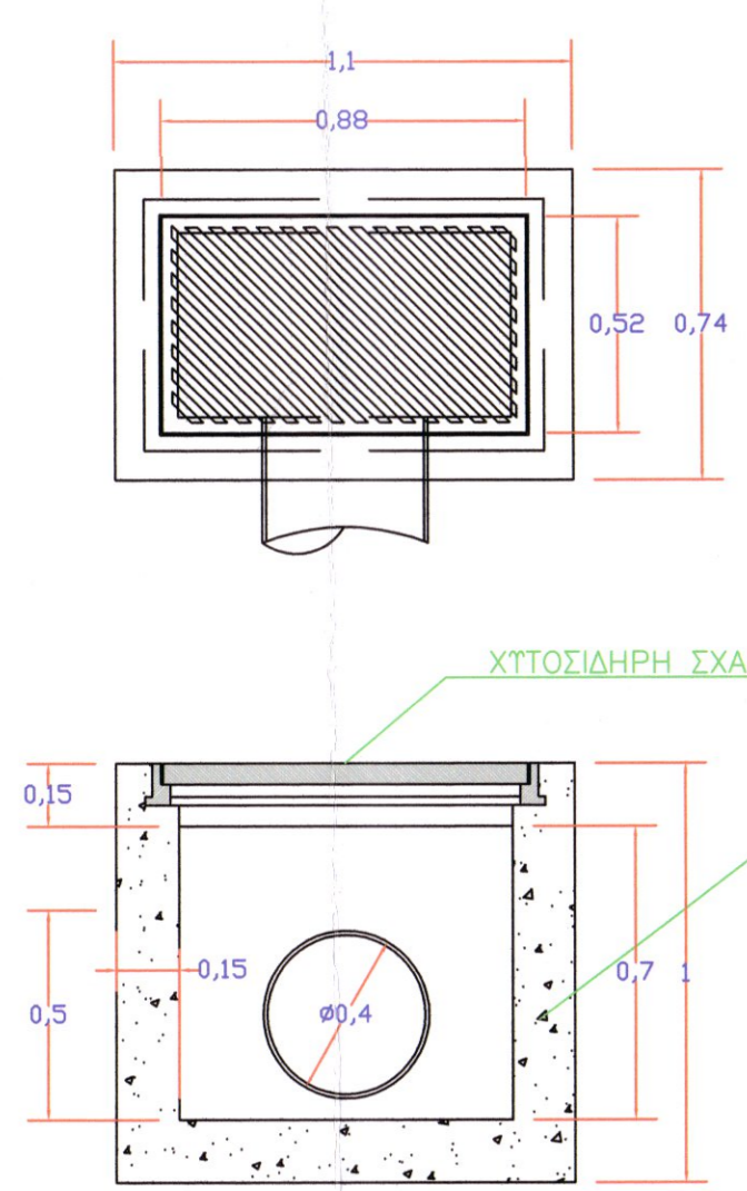
ΤΥΠΙΚΟ ΦΡΕΑΤΙΟ ΥΔΡΟΣΥΛΛΟΓΗΣ
